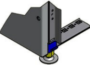
Höhenverstellfuß M12x35
