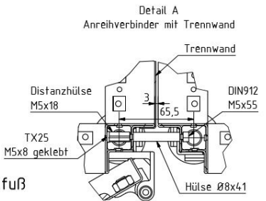
Anreihverbinder + Maße bei IS1
